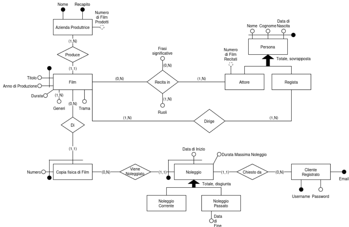
Figura 1: Schema Entità-Relazioni
