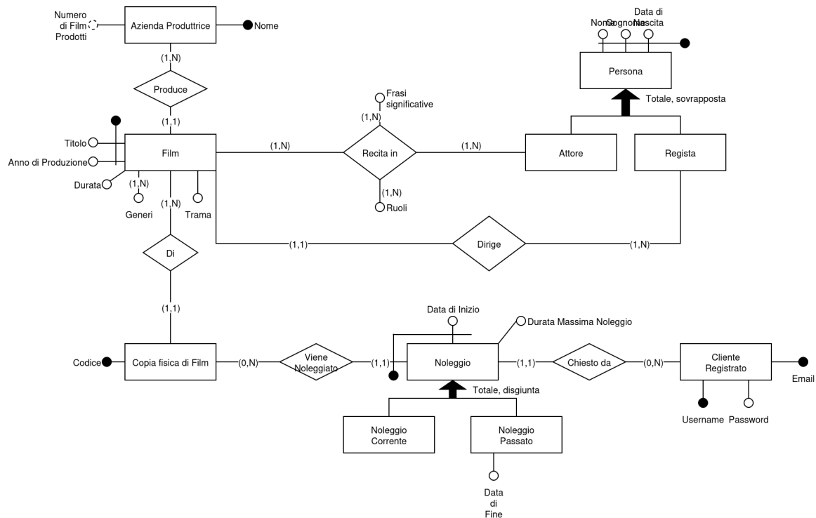
Figura 1: Schema Entità-Relazioni
