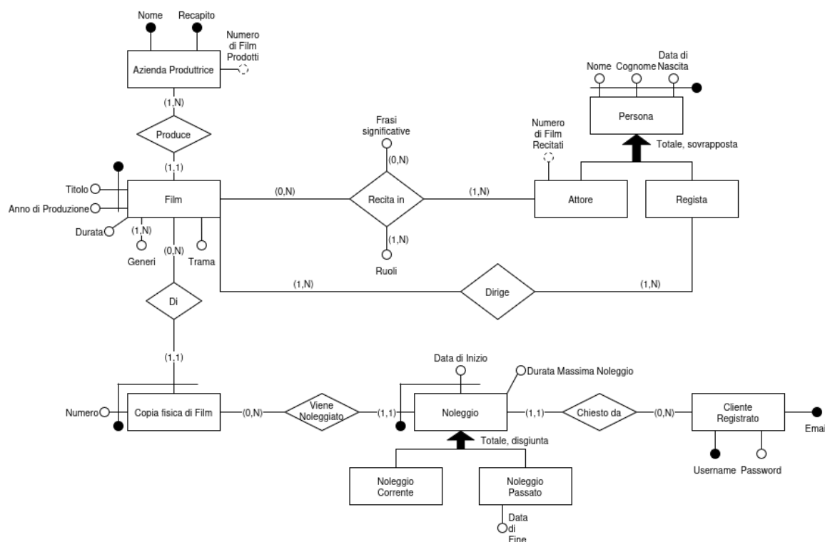
Figura 1: Schema Entità-Relazioni
