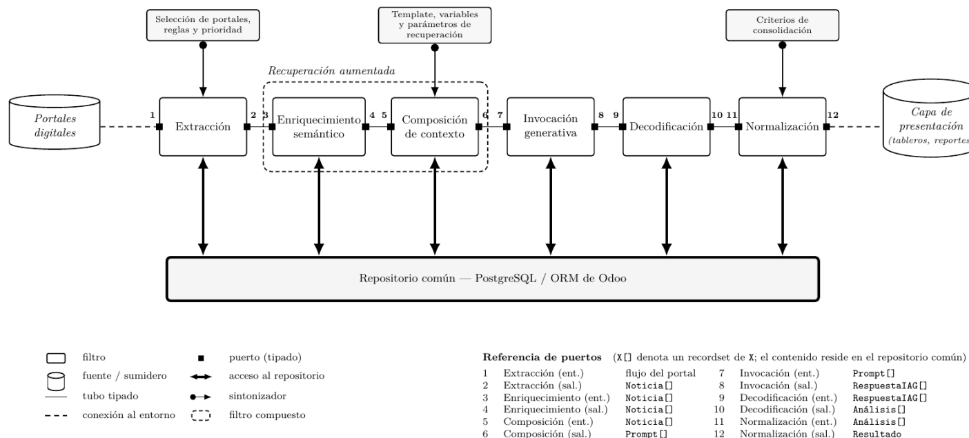
Figura 3.1: Diagrama canónico del framework propuesto como sistema de Tubos y Filtros. La fuente son los portales digitales de noticias y el sumidero es la capa de presentación de resultados (tableros y reportes). Los filtros se comunican mediante tubos tipados que transportan recordsets —conjuntos de referencias a registros—, cuyos puertos se numeran y se detallan en la tabla de referencia inferior; el contenido completo de esos registros reside en el repositorio común. Siguiendo la convención del estilo, las conexiones al entorno se representan con línea discontinua y los tubos entre filtros con línea continua —ambos sin punta, dado que el flujo se asume de izquierda a derecha—, en tanto que los sintonizadores —modulares, uno por filtro— se grafican con flecha originada en un círculo y el acceso al repositorio con flecha bidireccional. El recuadro de trazo discontinuo que engloba los filtros de Enriquecimiento semántico y Composición de contexto indica que ambos conforman un filtro compuesto, denominado Recuperación aumentada.
