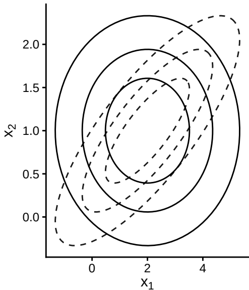
Kullback–Leibler
