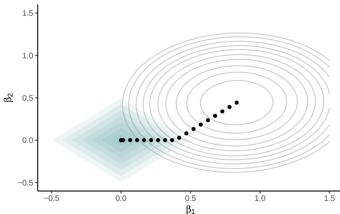
FIGURE 3.9 – Courbes de contour du critère de l'erreur quadratique moyenne (ellipses) et fonction de pénalité (losanges) pour différentes valeurs de \lambda . Les points dénotent des solutions différentes et intersectent les contours du losange.
