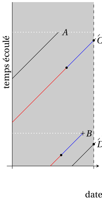
FIGURE 5.6 – Diagramme de Lexis avec trajectoires. Pour ajuster le modèle, on peut casser la contribution d’une observation en segments : considérons un seul changement survenant au temps t_c . Pour le premier segment, on enregistre t_c comme valeur maximale (censure à droite), tandis que pour la deuxième portion, l’observation est tronquée à gauche à partir de t_c .
