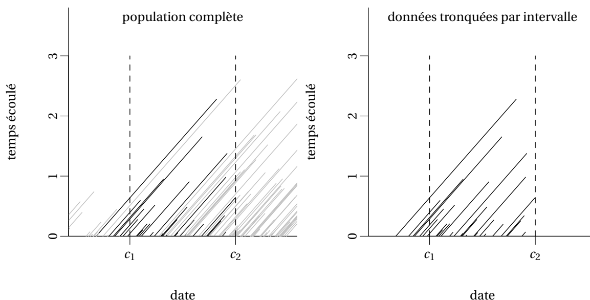
FIGURE 5.2 – Diagramme de Lexis illustrant la troncature par intervalle.
