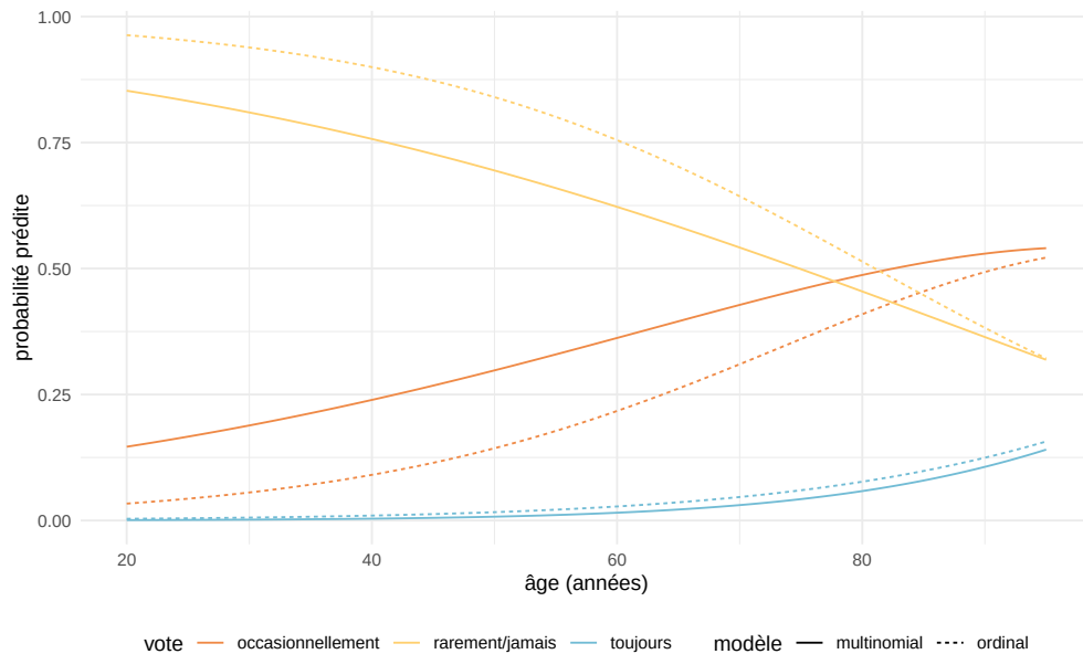
FIGURE 4.11 – Probabilités prédites pour chaque modalité selon le modèle de régression multinomiale logistique et le modèle de régression ordinales à cotes proportionnelles selon l'âge.
