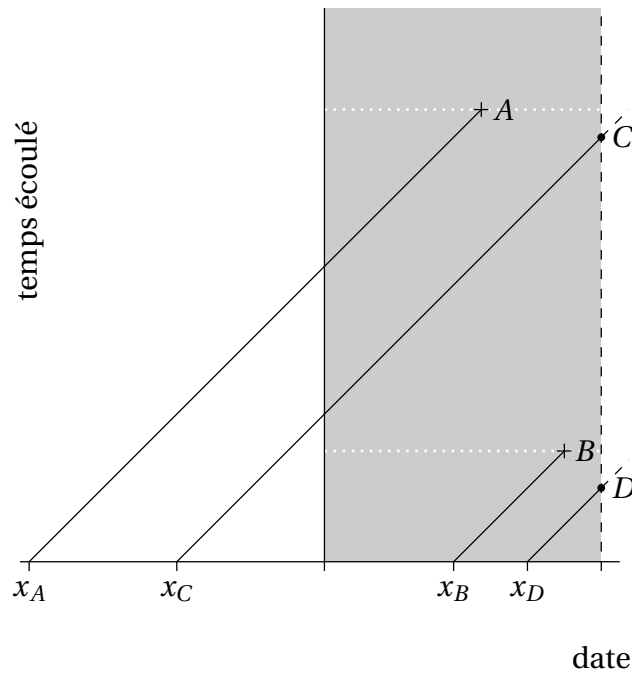
FIGURE 5.1 – Diagramme de Lexis pour données tronquées à gauche (A et C) et censurées à droite (C et D).
