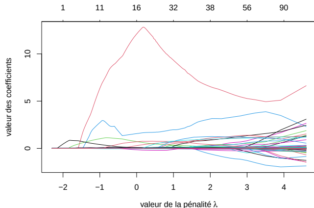
Figure 1: Valeur des coefficients du modèle en fonction de la pénalité (avec nombre de coefficients non-nuls sur le dessus).
