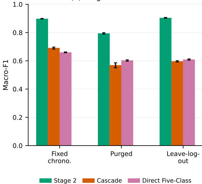
(b) Diagnostic Macro-F1
