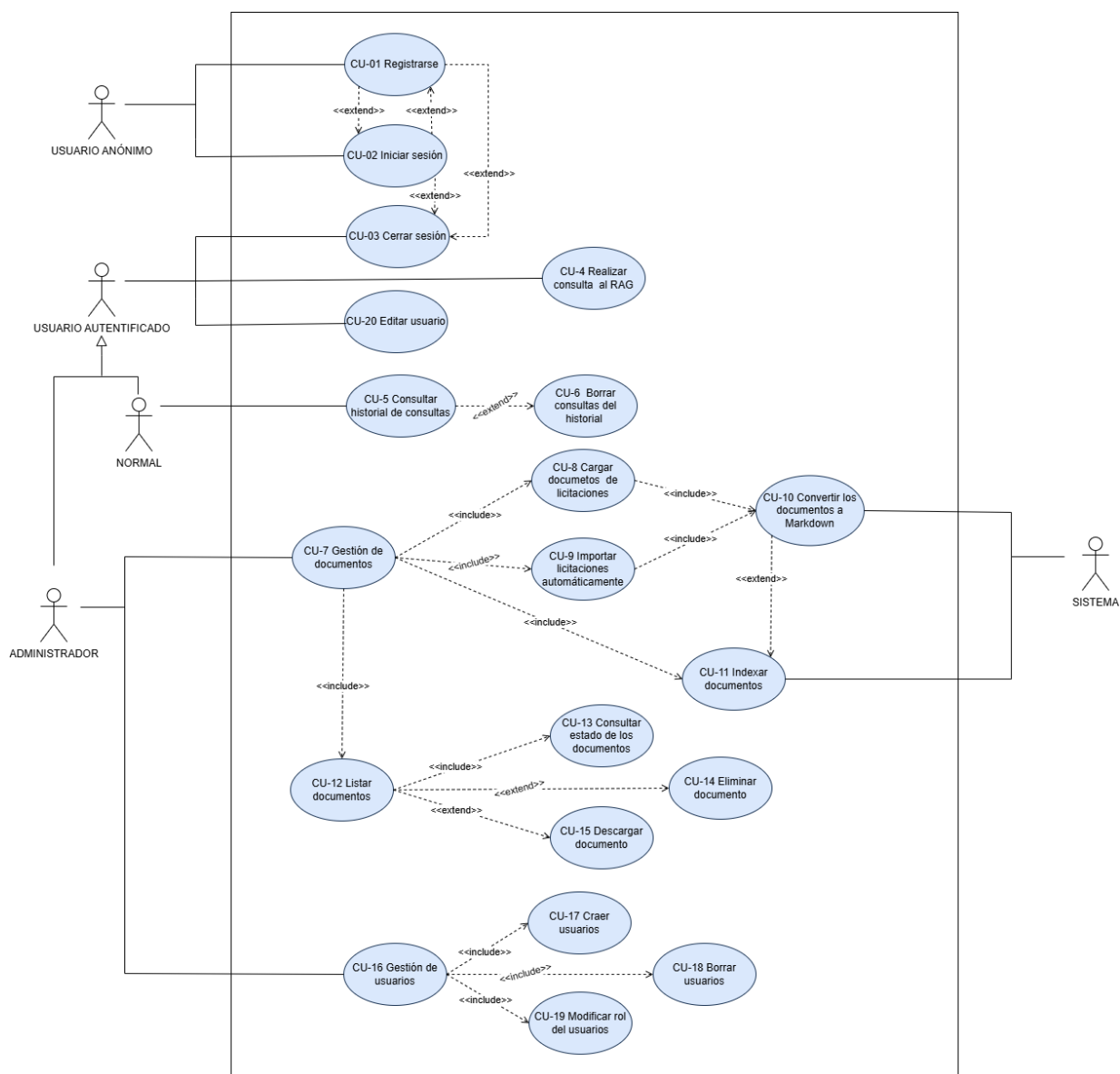
Figura B.1: Diagrama general de casos de uso.
