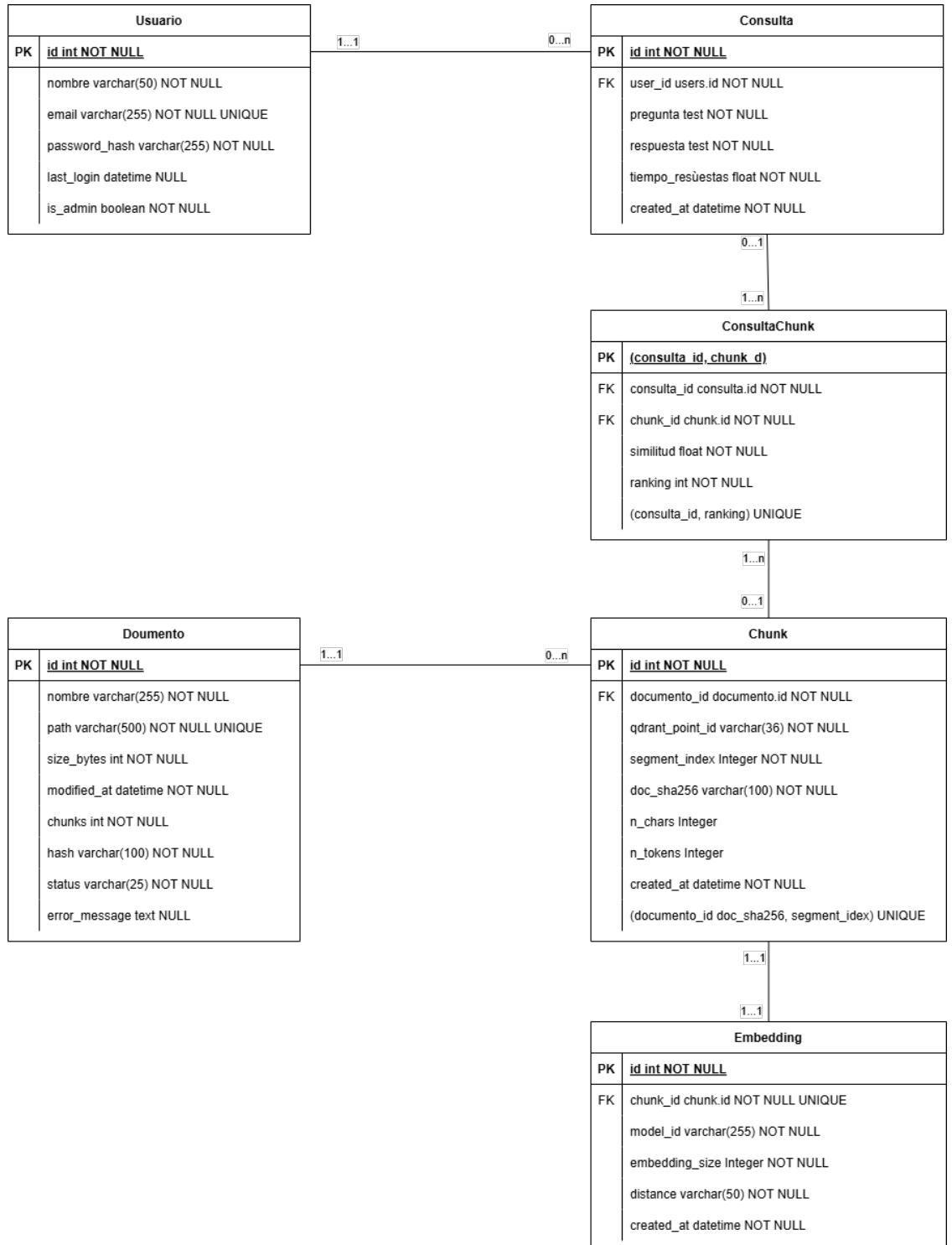
Figura C.2: Diagrama relacional.
