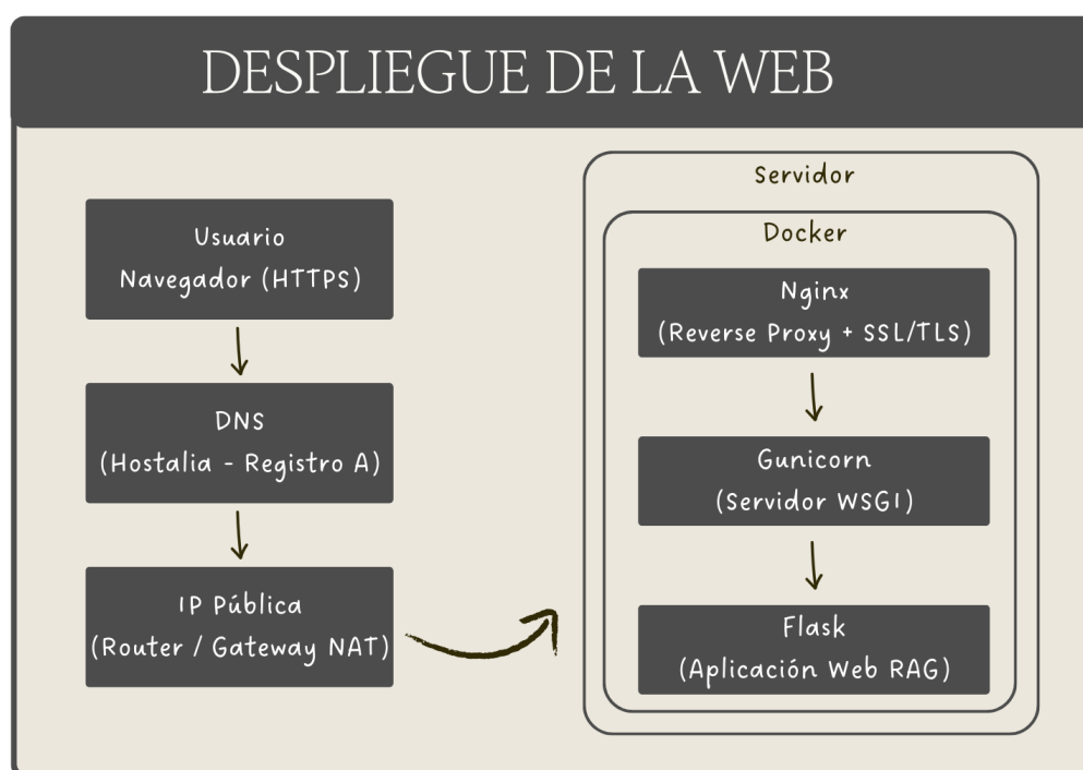
Figura 4.4: Relación entre las herramientas utilizadas para desplegar la aplicación web .
