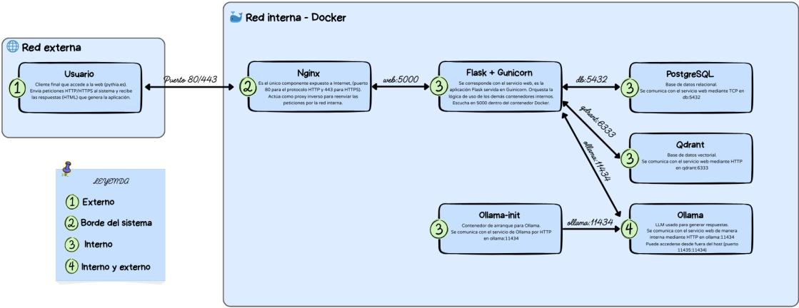
Figura C.3: Diagrama de la comunicación entre los principales componentes del sistema.
