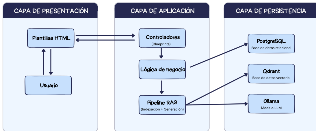
Figura C.5: Diagrama de la arquitectura lógica del sistema.
