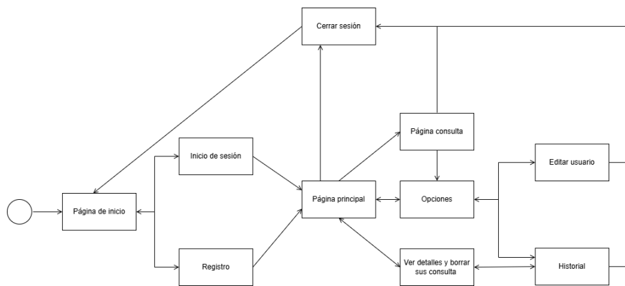
Figura C.16: Diagrama de navegabilidad por la aplicación para el usuario normal.
