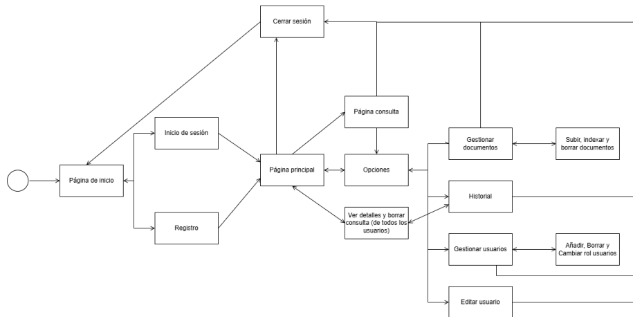
Figura C.15: Diagrama de navegabilidad por la aplicación para el administrador.
