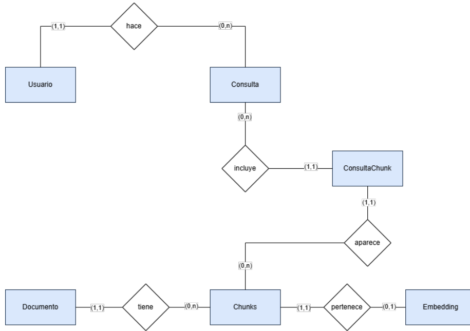
Figura C.1: Diagrama Entidad/Relación.
