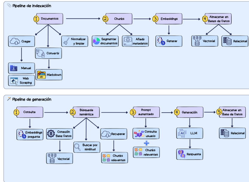
Figura C.7: Diagrama de la arquitectura del modelo RAG .
