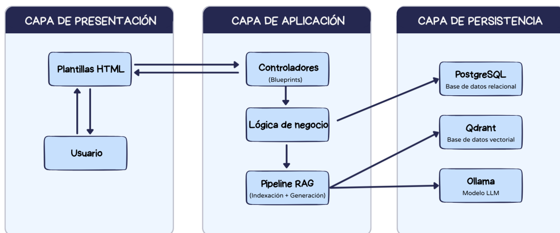
Figura C.5: Arquitectura cliente-servidor multicapa.
