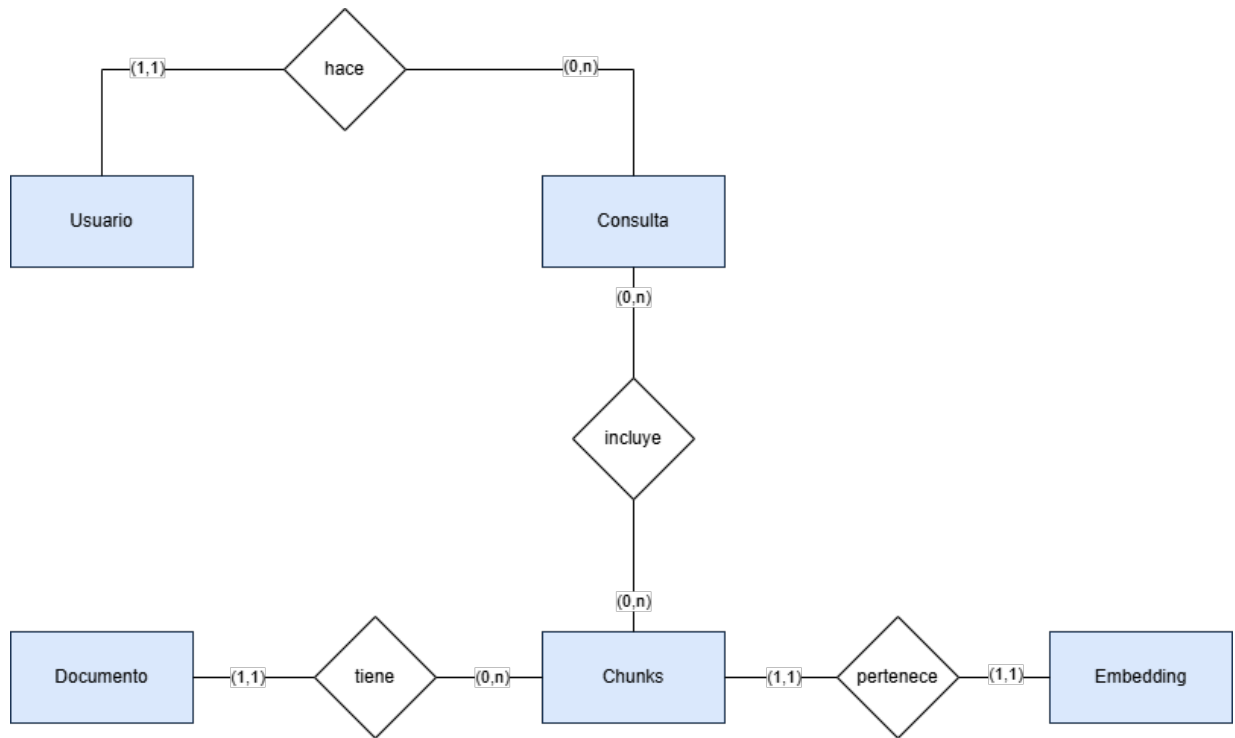
Figura C.1: Diagrama Entidad/Relación.
