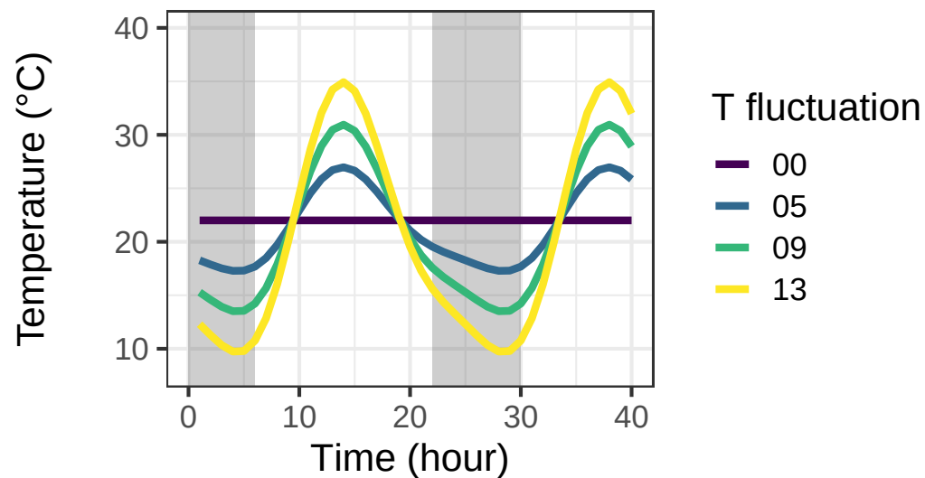
E) expt 5. hot days
