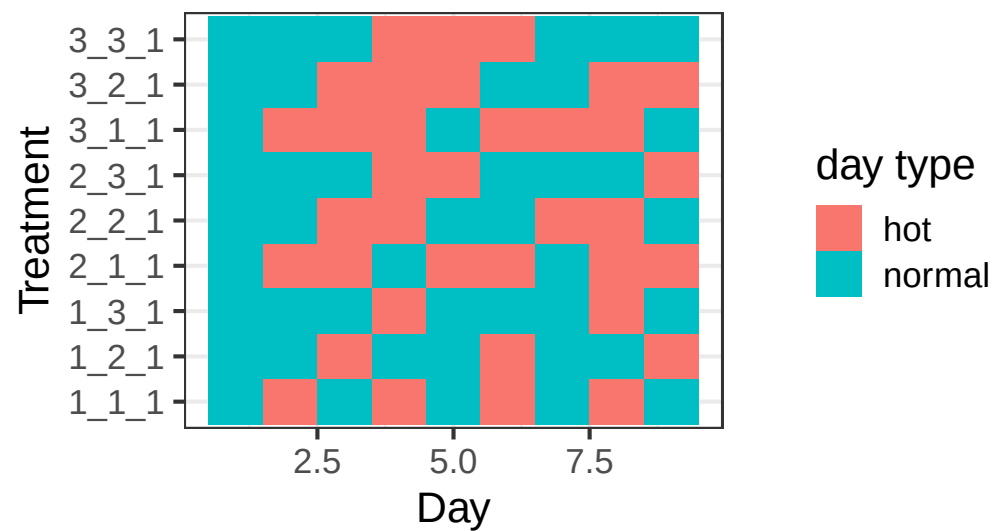
E) expt 5. hot days
