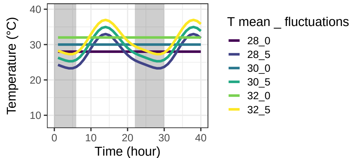
F) expts 6 & 7. heat waves
