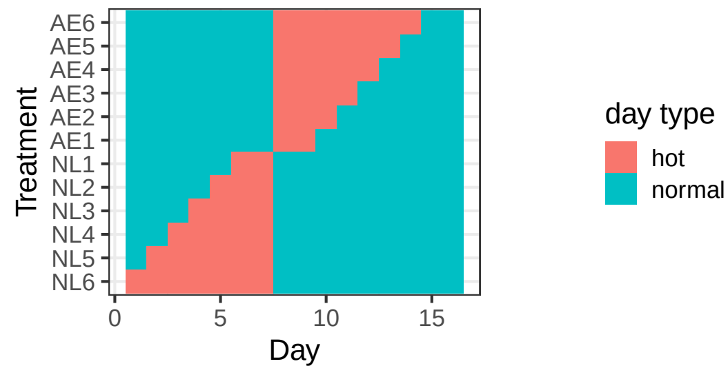
F) expts 6 & 7. heat waves
