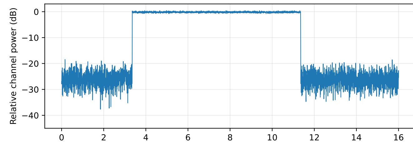
transitions-none
