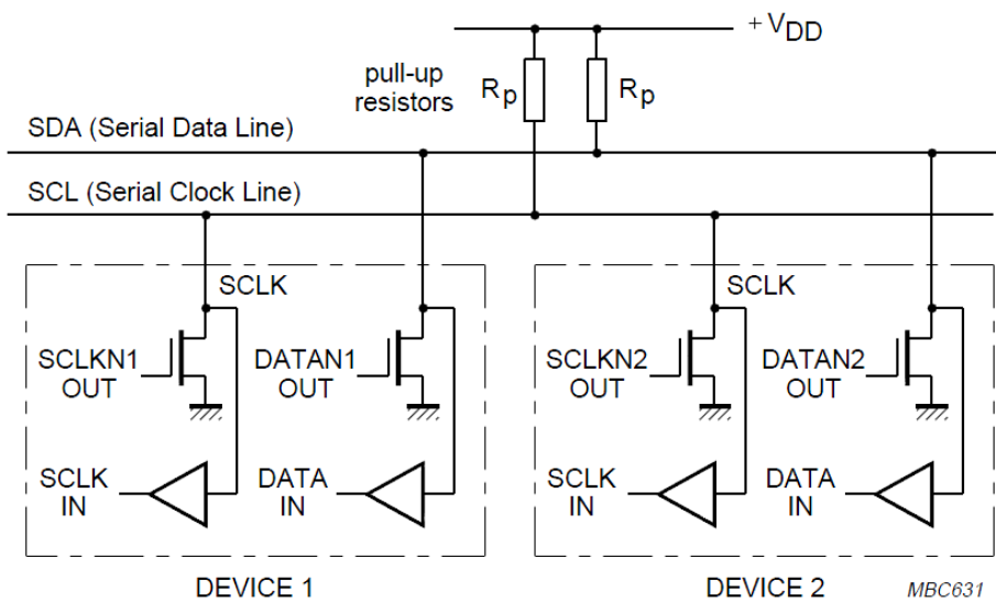
图 9 IIC 串行通信标准的连接方式
