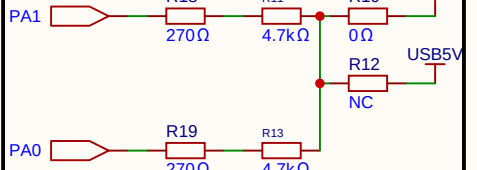
开漏式IO的上拉电阻
