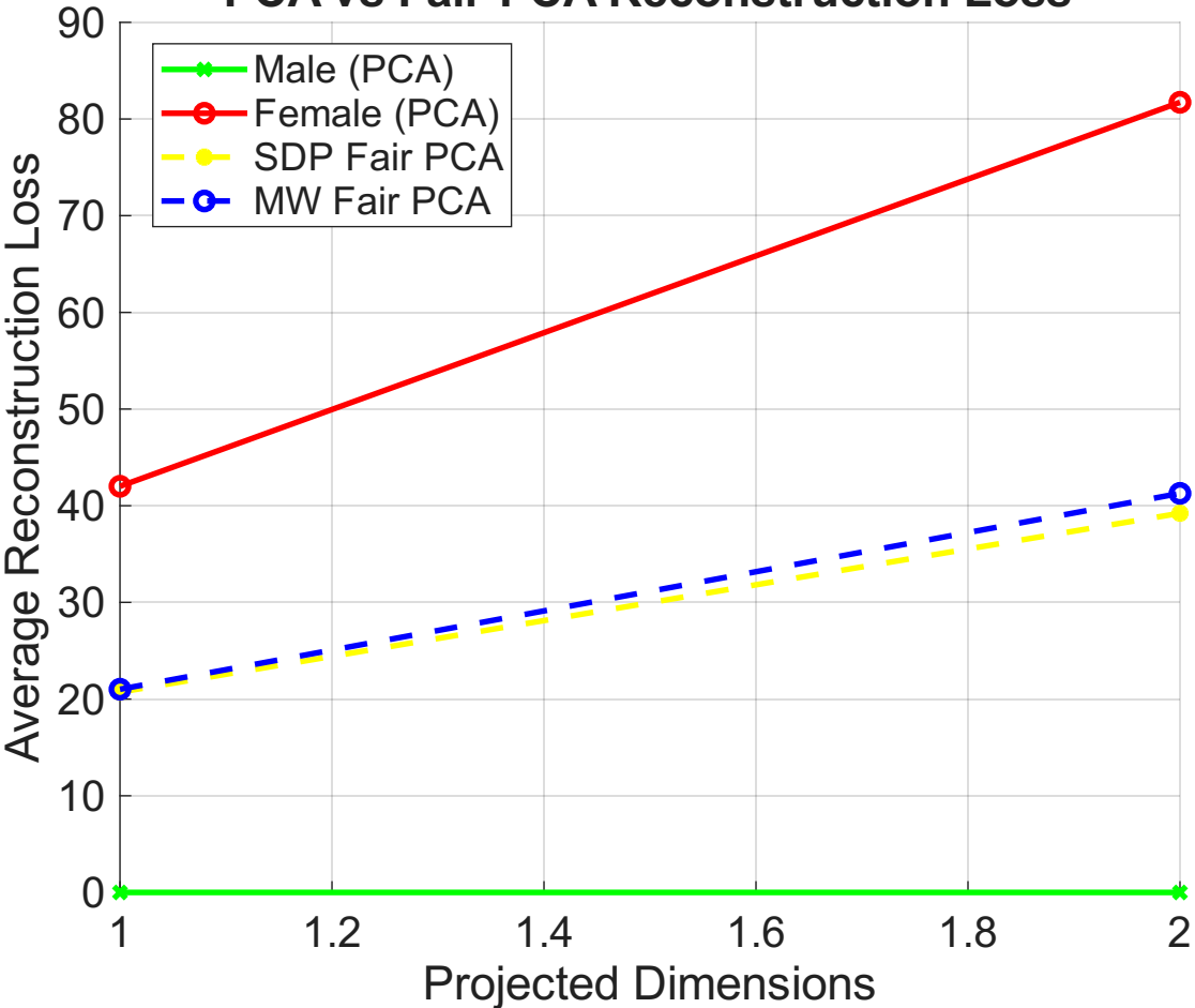
PCA vs Fair-PCA Reconstruction Loss
