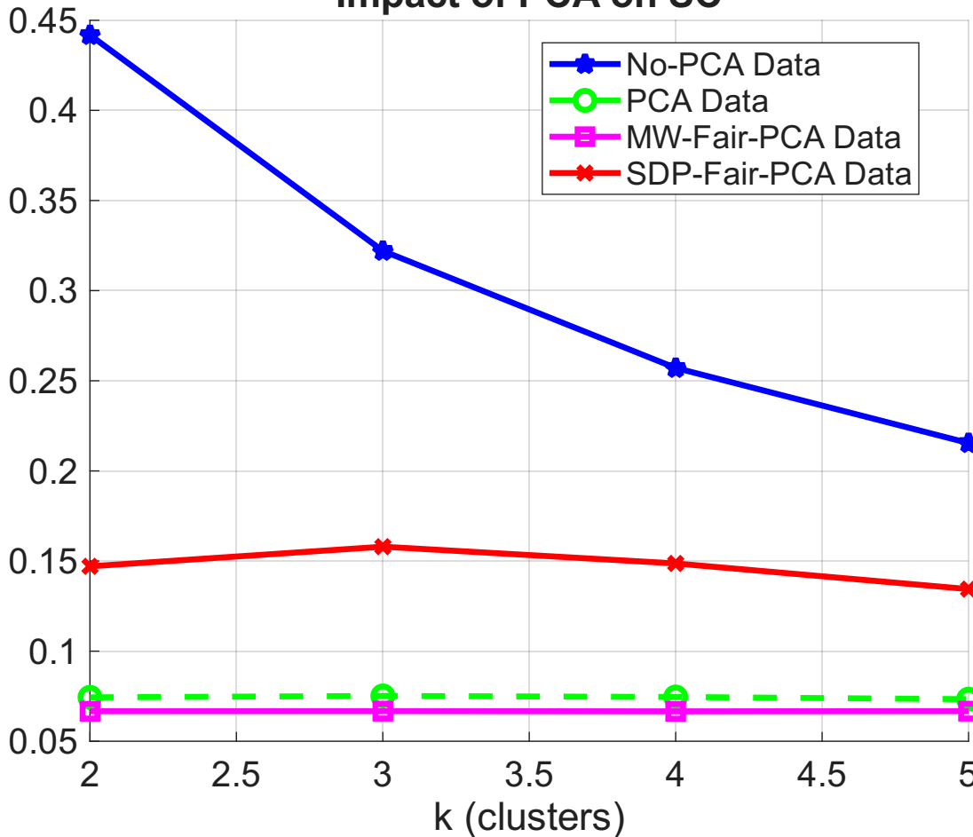
Impact of PCA on SC
