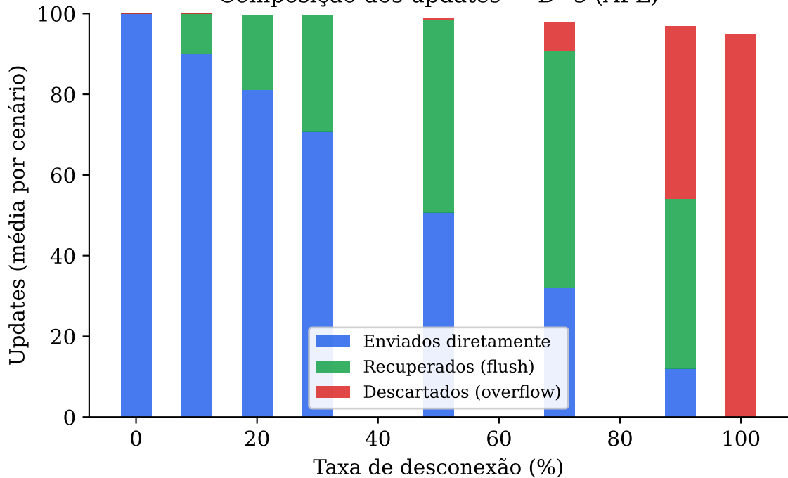
Composição dos updates — B=5 (AFL)
