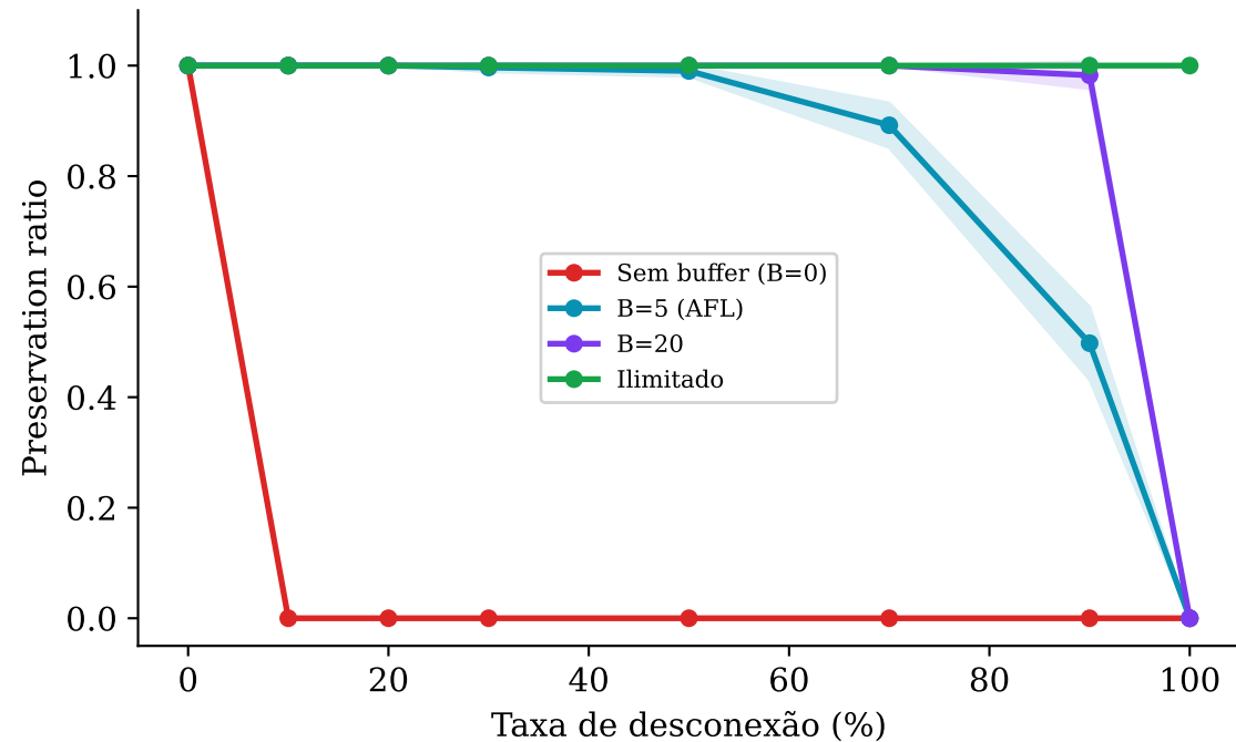
Preservação vs desconexão, por tamanho de buffer
