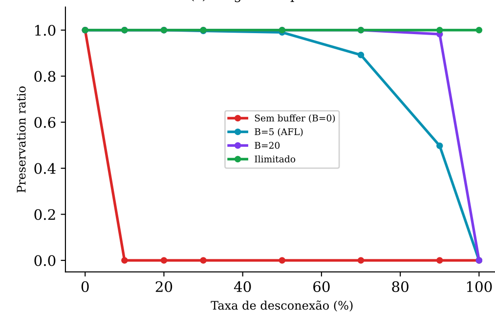
(c) Ring buffer por tamanho
