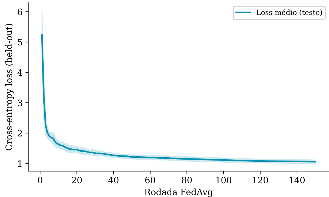
Loss de validação por rodada
