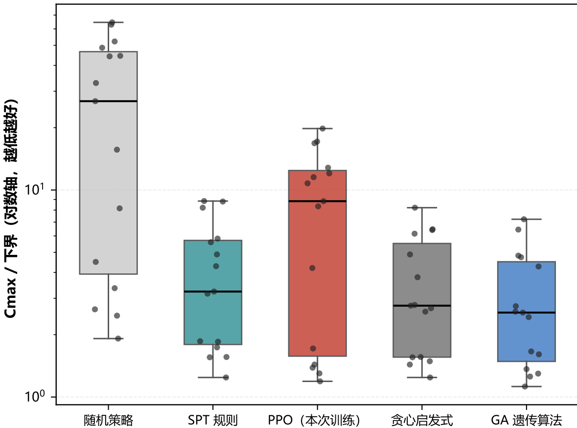
(a) 绝对排程质量分布 (15 个实例)
