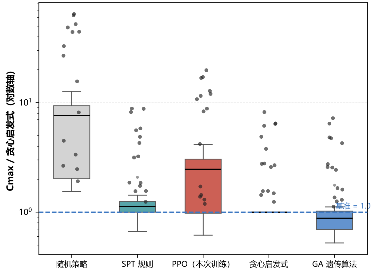
(b) 相对贪心启发式的比率
