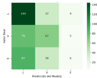
Figura 3. Matriz de confusión Naive Bayes manual
