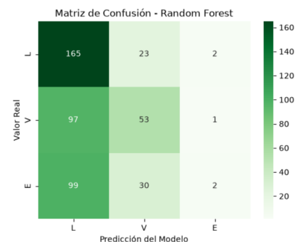
Figura 5. Matriz de confusión Random Forest scikit learn
