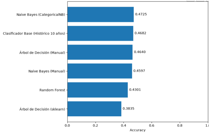
Figura 6. Accuracy de los modelos ajustados
