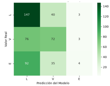
Figura 4. Matriz de confusión del ajuste Naive Bayes Scikit Learn
