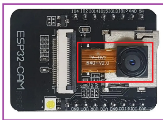
Módulo ESP32-CAM
