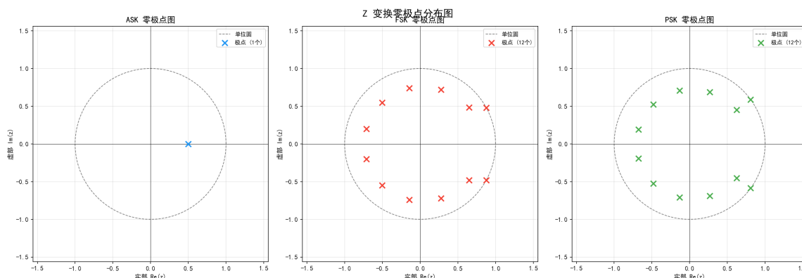
图 5: Z 变换零极点分布 (AR 模型建模)
