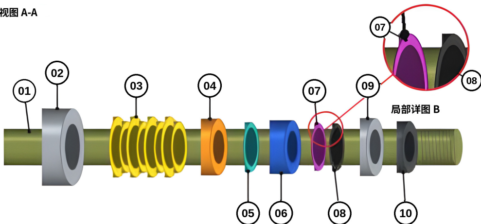
芯轴组件爆炸图
