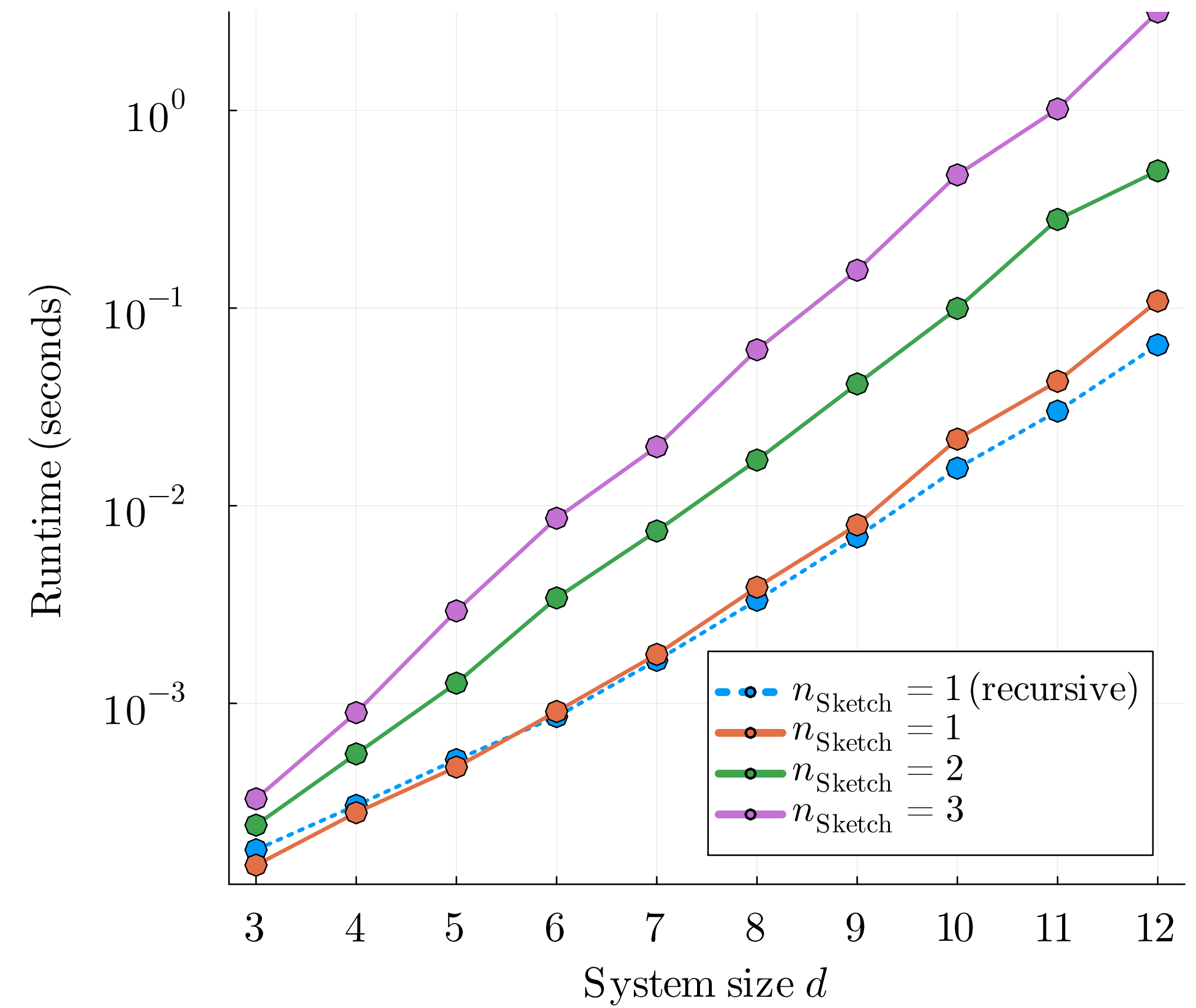
(d) Runtime vs. System size d
