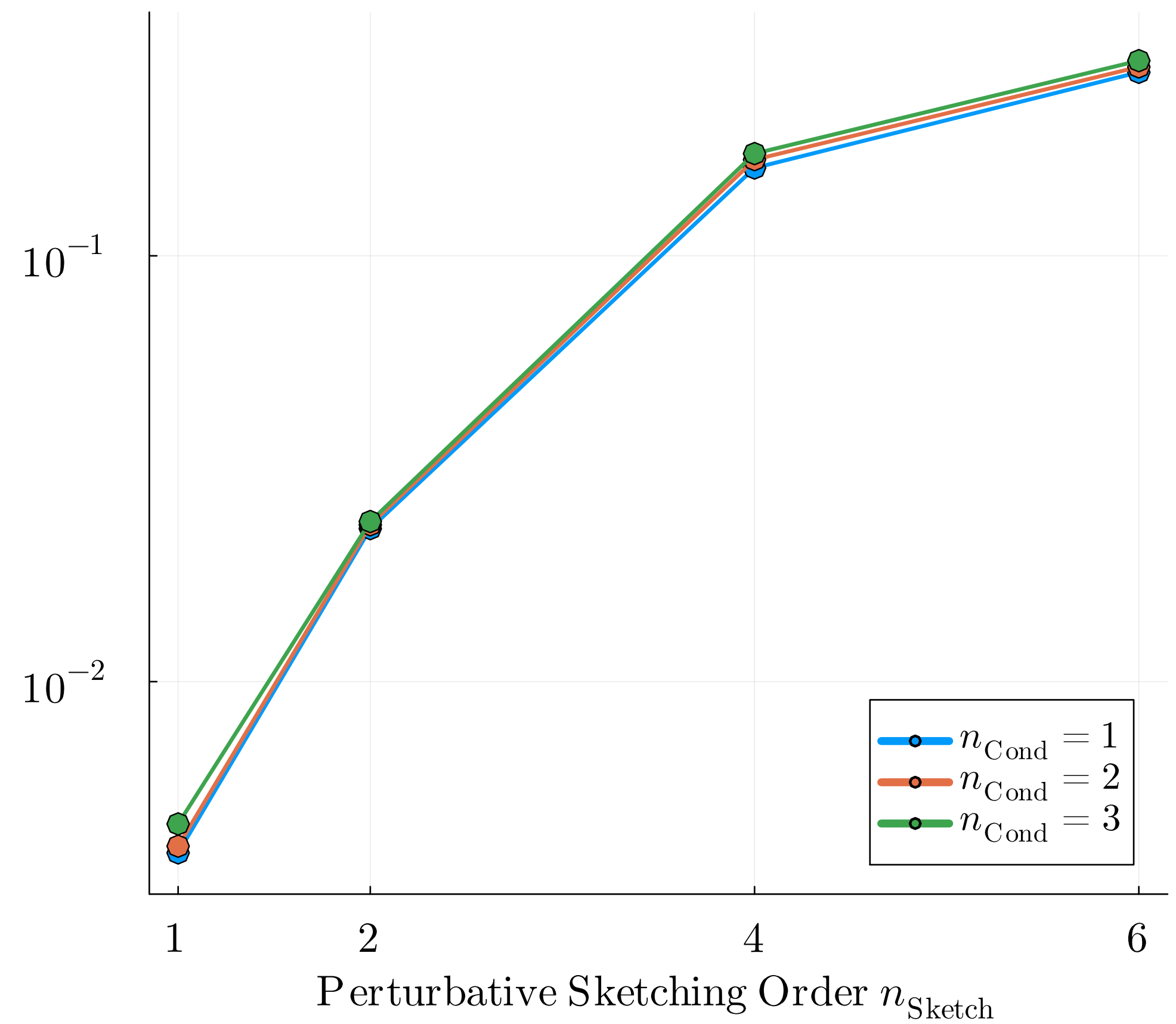
(d) Runtime (s)
