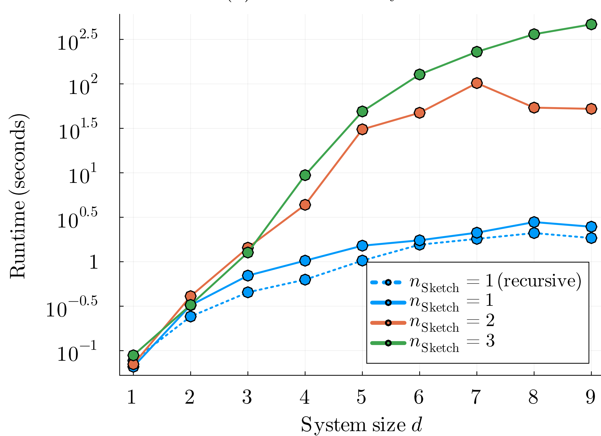
(d) Runtime vs. System size d
