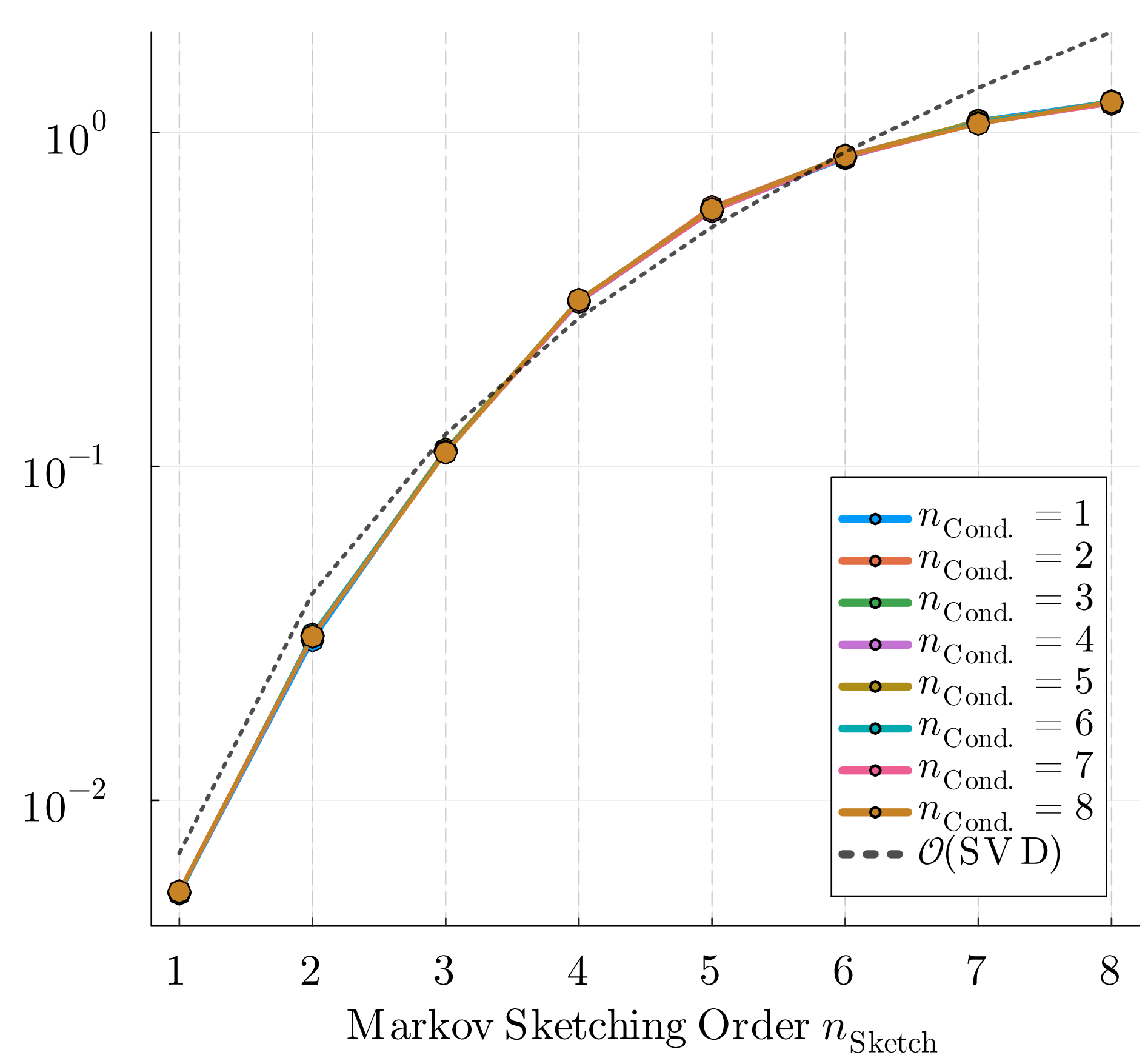
(d) Runtime (s)
