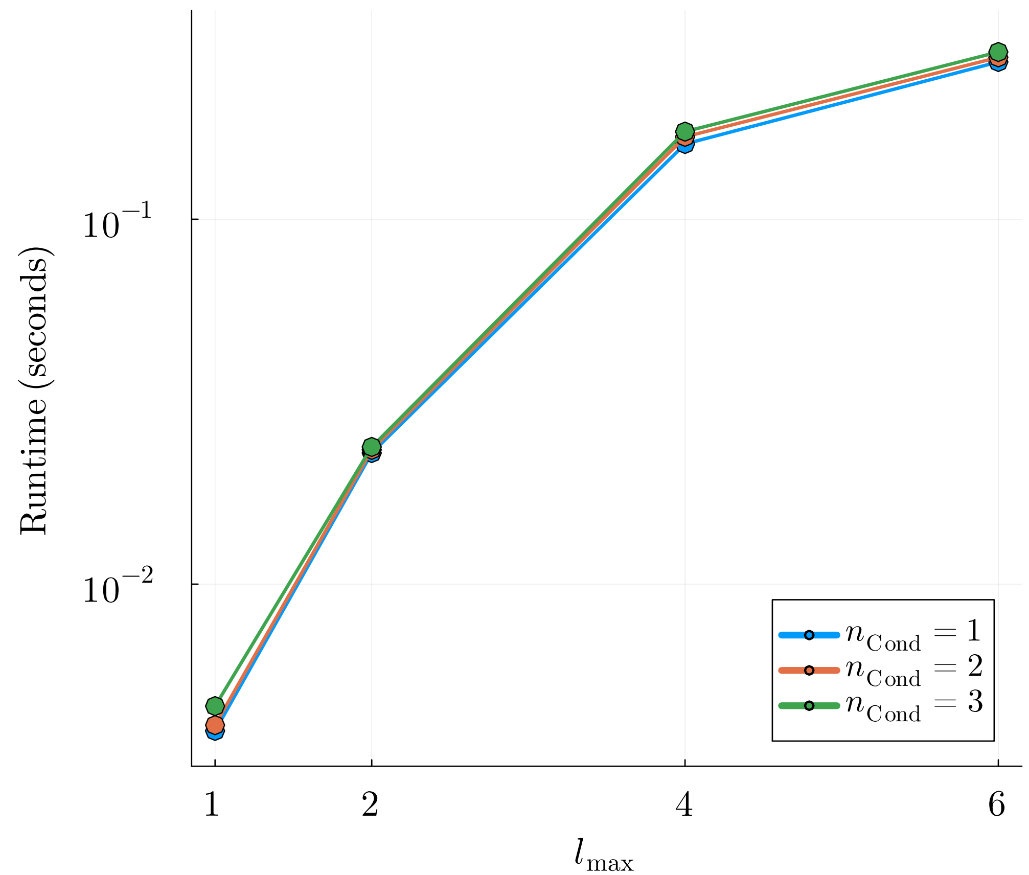
(d) Runtime vs. max. cardinality l_{\text{max}} = |\mathcal{S}|
