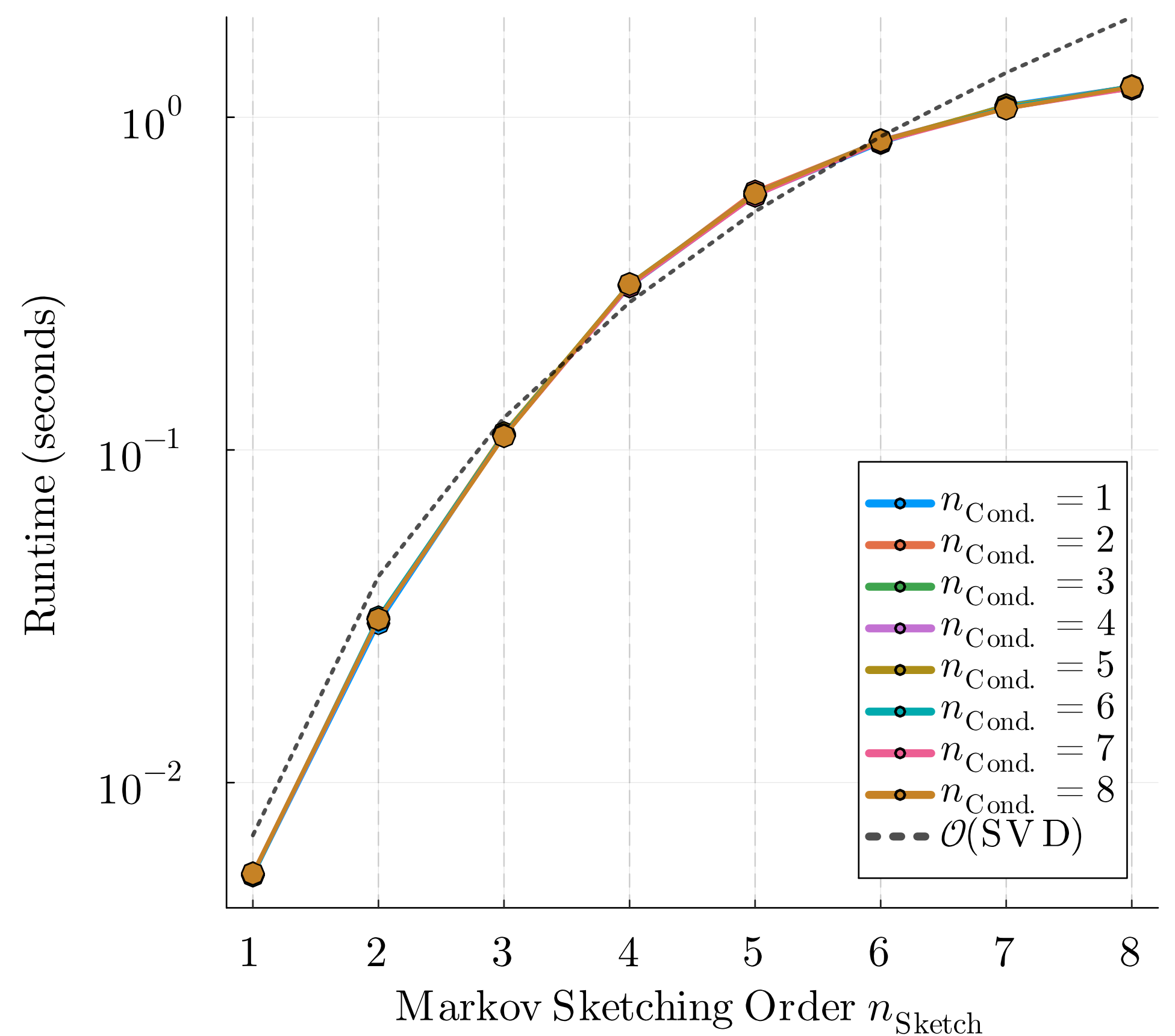
(d) Runtime vs. Markov Sketching Order n_{\text{Sketch}}
