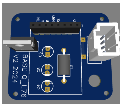
FIGURA 3.8. Modelo 3D del adaptador L76.
