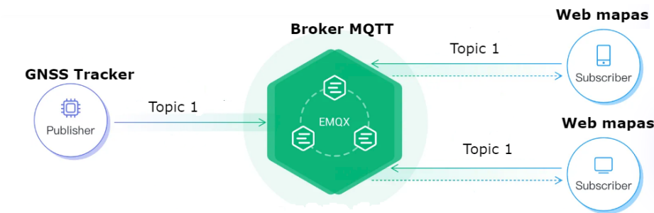
FIGURA 3.14. Arquitectura MQTT 1 .
