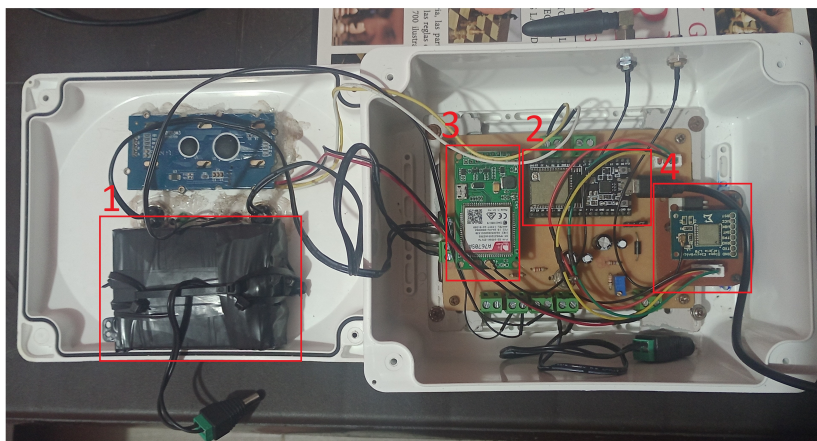
FIGURA 4.4. Vista real de los componentes del hardware (interior).
