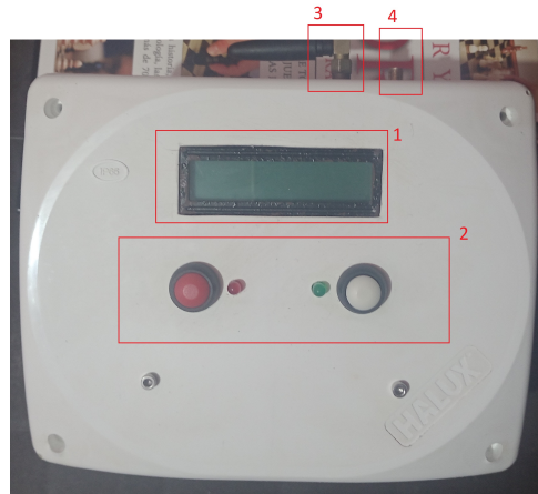
FIGURA 4.3. Vista real de los componentes del hardware (exterior).
