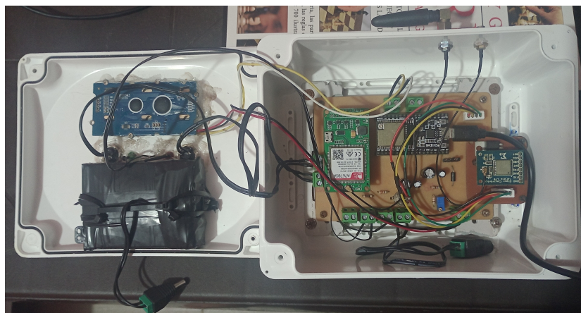
FIGURA 4.2. Resultado final del hardware desarrollado (interior).
