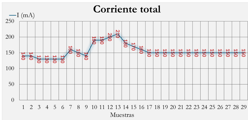
FIGURA 4.6. Gráfico de la muestras tomadas en la medición de corriente.
