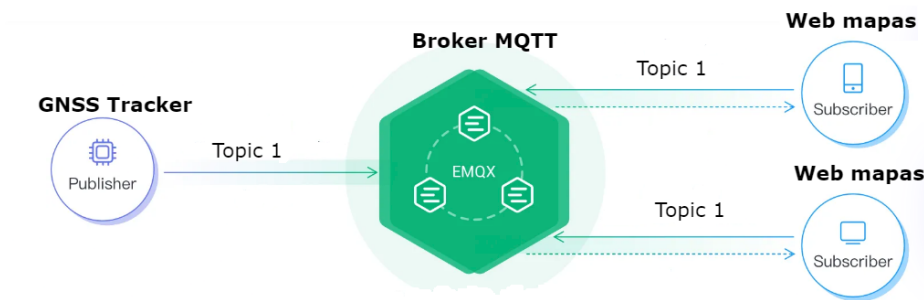
FIGURA 3.14. Arquitectura MQTT 1 .
