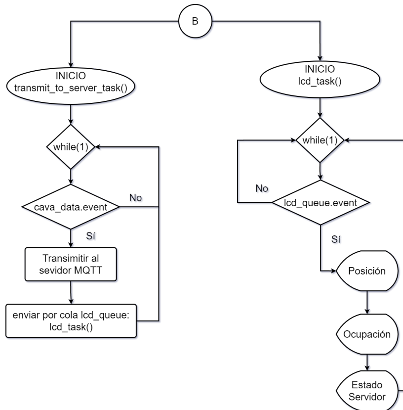
FIGURA 3.13. Diagrama de flujo del firmware (parte 3).
