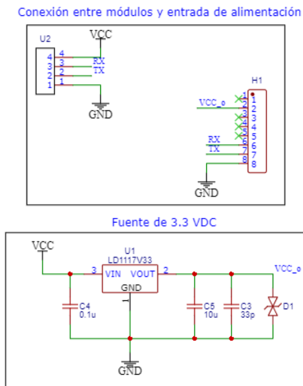
FIGURA 3.6. Esquemático del adaptador L76.
