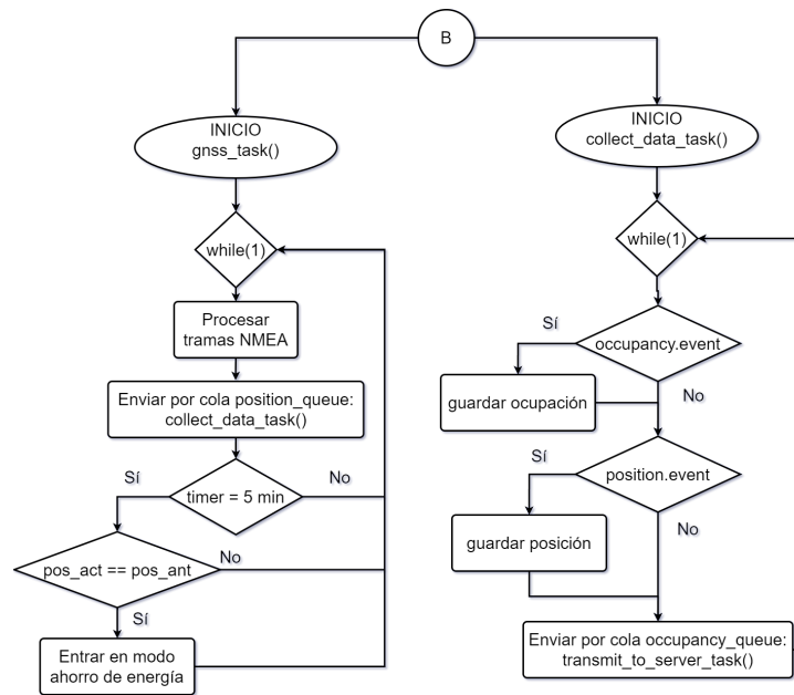
FIGURA 3.12. Diagrama de flujo del firmware (parte 2).
