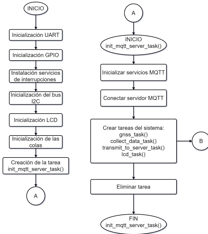
FIGURA 3.11. Diagrama de flujo del firmware (parte 1).
