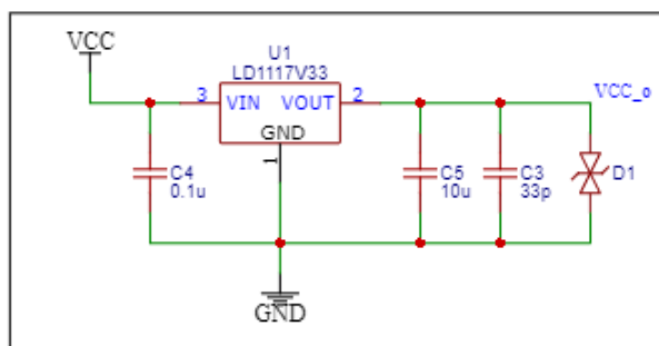
Fuente de 3.3 VDC
