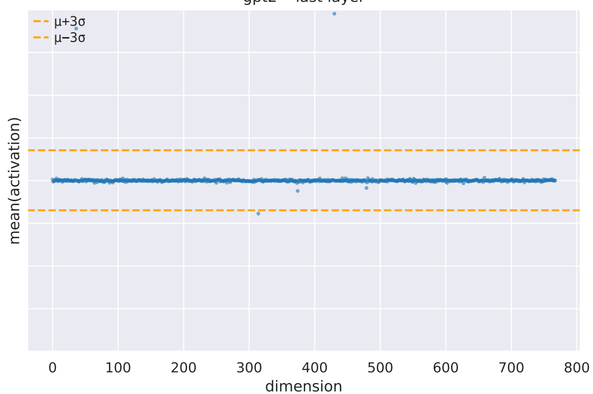
gpt2 • last layer
