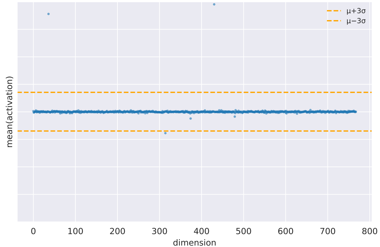
gpt2 • last layer
