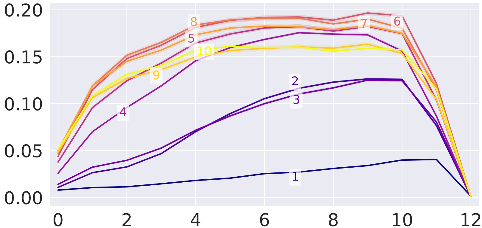
GPT
