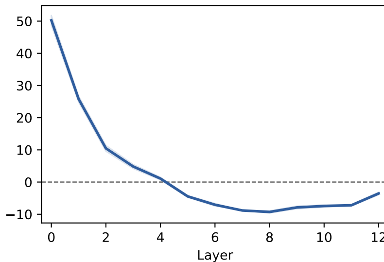
Linear ID
