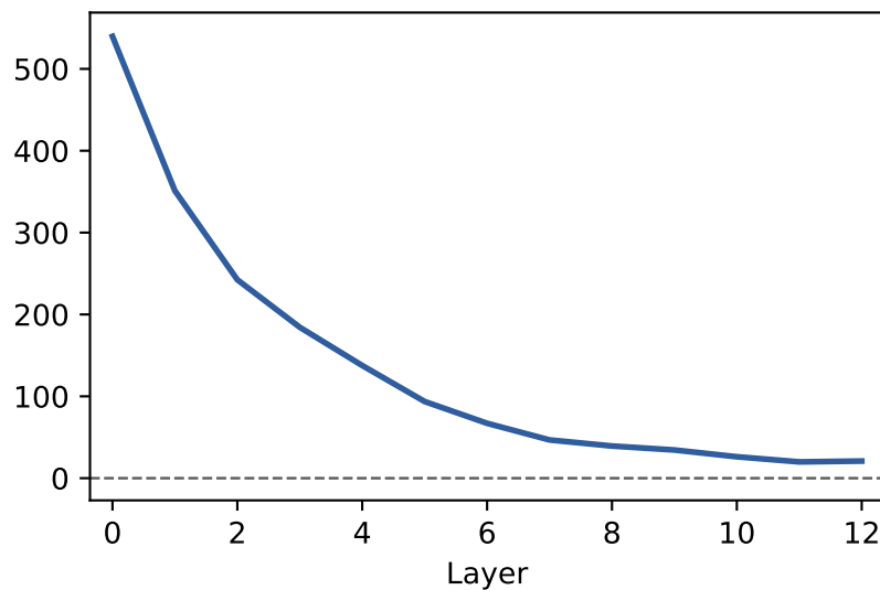
Linear ID
