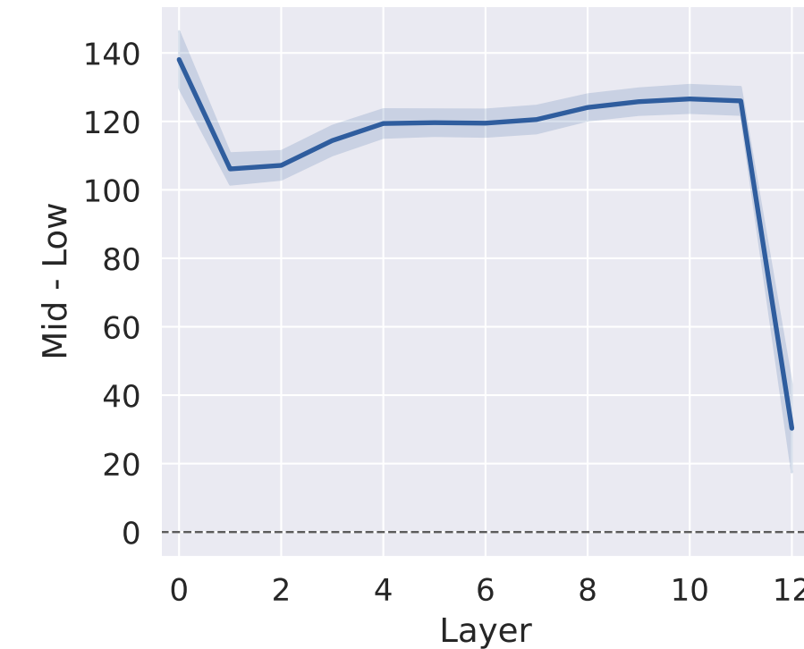
GPT Linear ID
