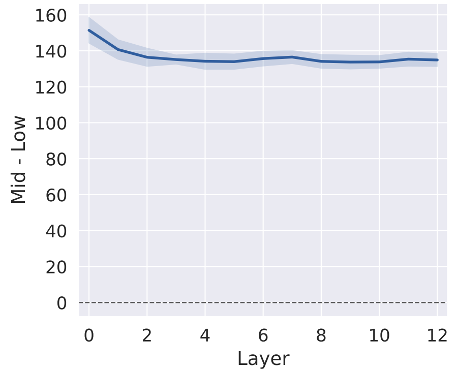
BERT Linear ID
