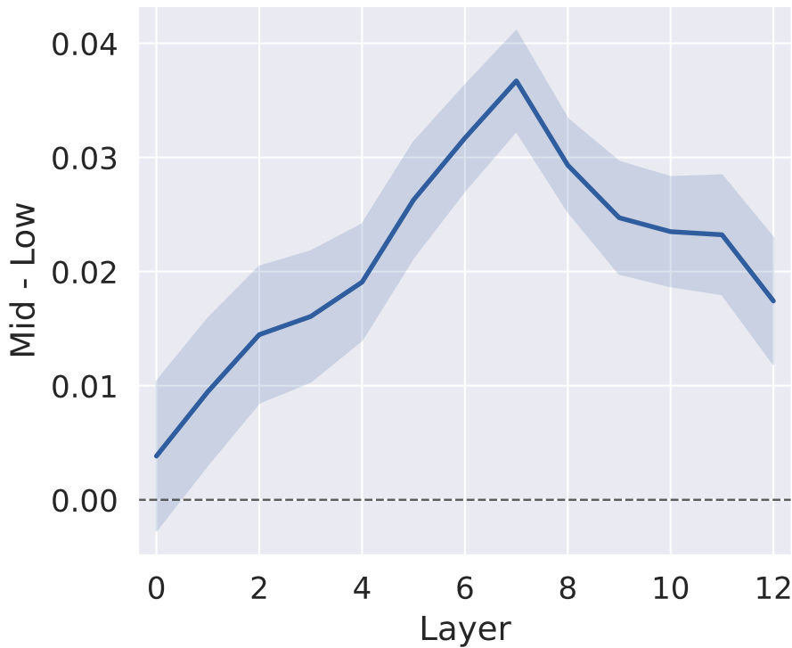
BERT IsoScore
