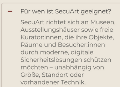
interaktive FAQ-Komponente
