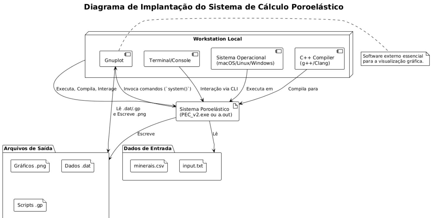
Figura 4.2: Diagrama de implantação
