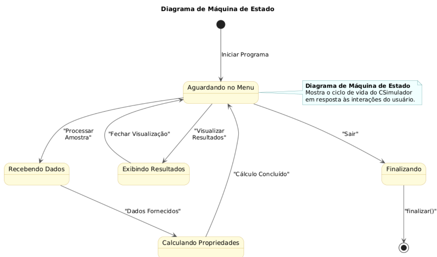
Figura 3.5: Diagrama de máquina de estado
