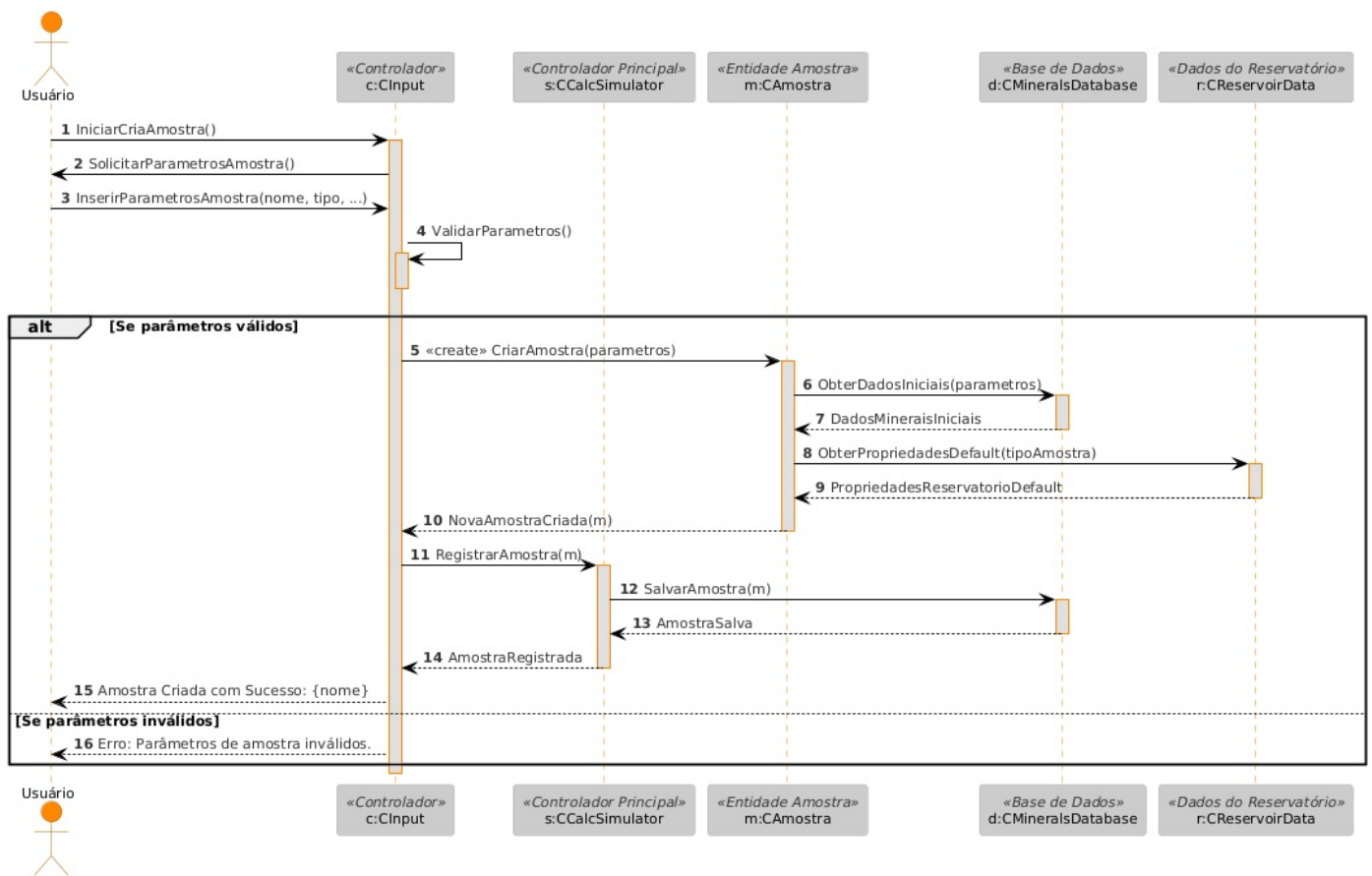
Figura 3.3: Diagrama de sequência específico
