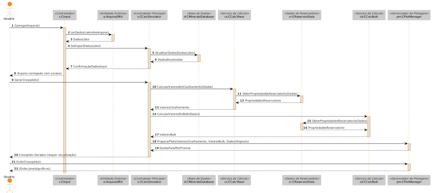
Figura 3.2: Diagrama de seqüência geral
