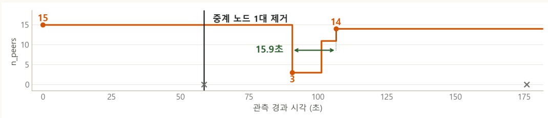
중계 노드 1대 제거 → 15.9초 만에 재구성 (2026-09-01 실측)
