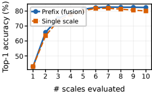
Oxford-Pets (text)
