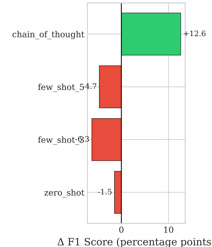
F1 Score
