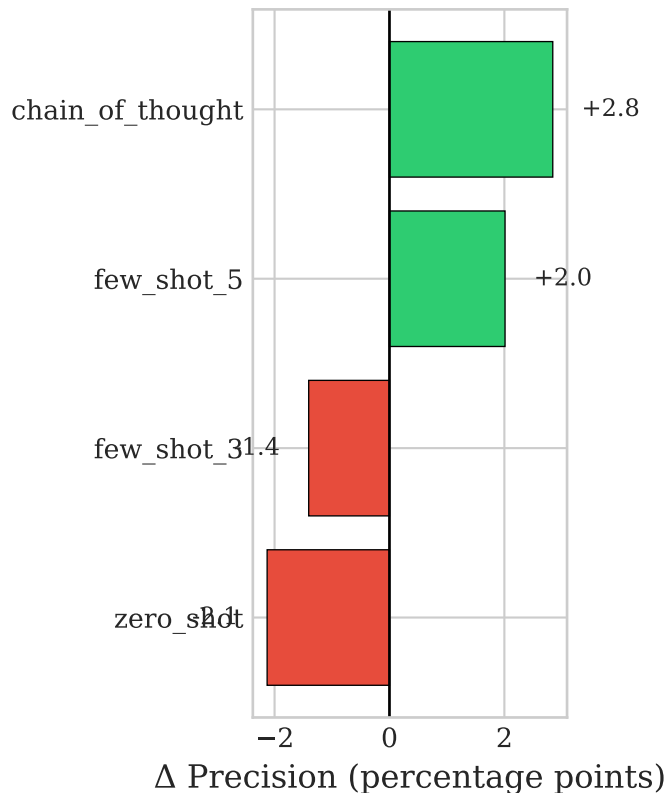
Precision
