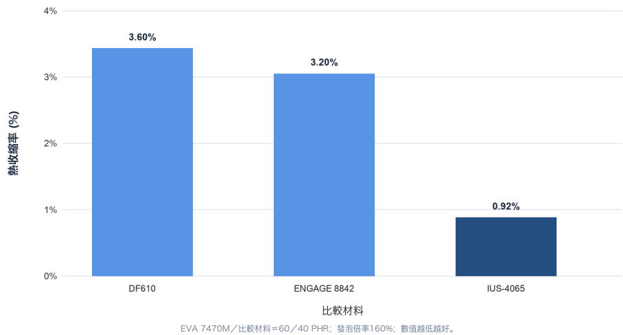
70° C / 40分鐘熱收縮率比較
