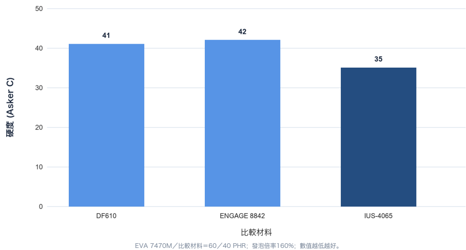
發泡成品硬度比較
