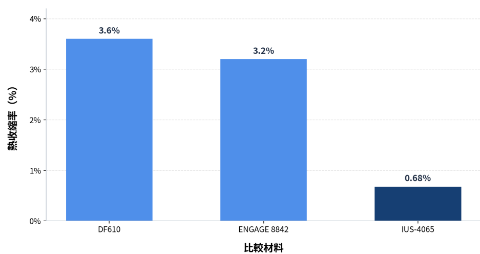
70°C／40分鐘熱收縮率比較
