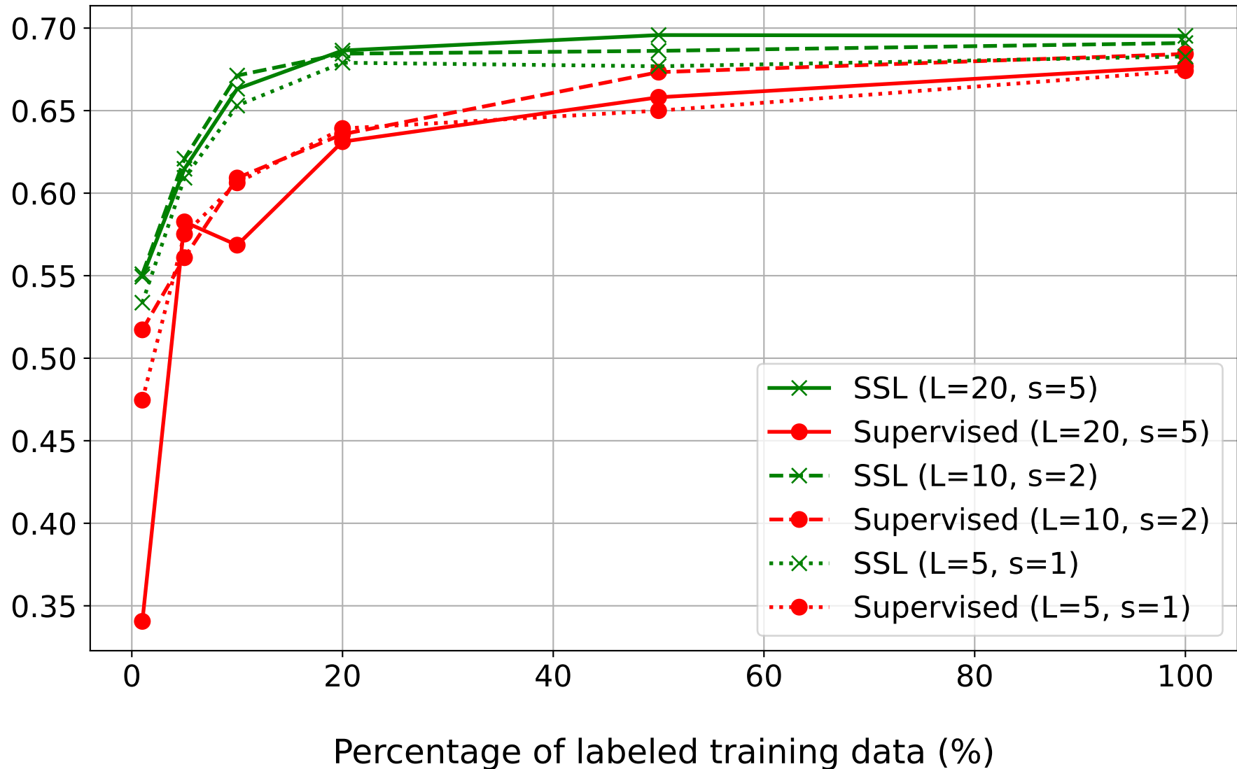
Macro F1 Score
