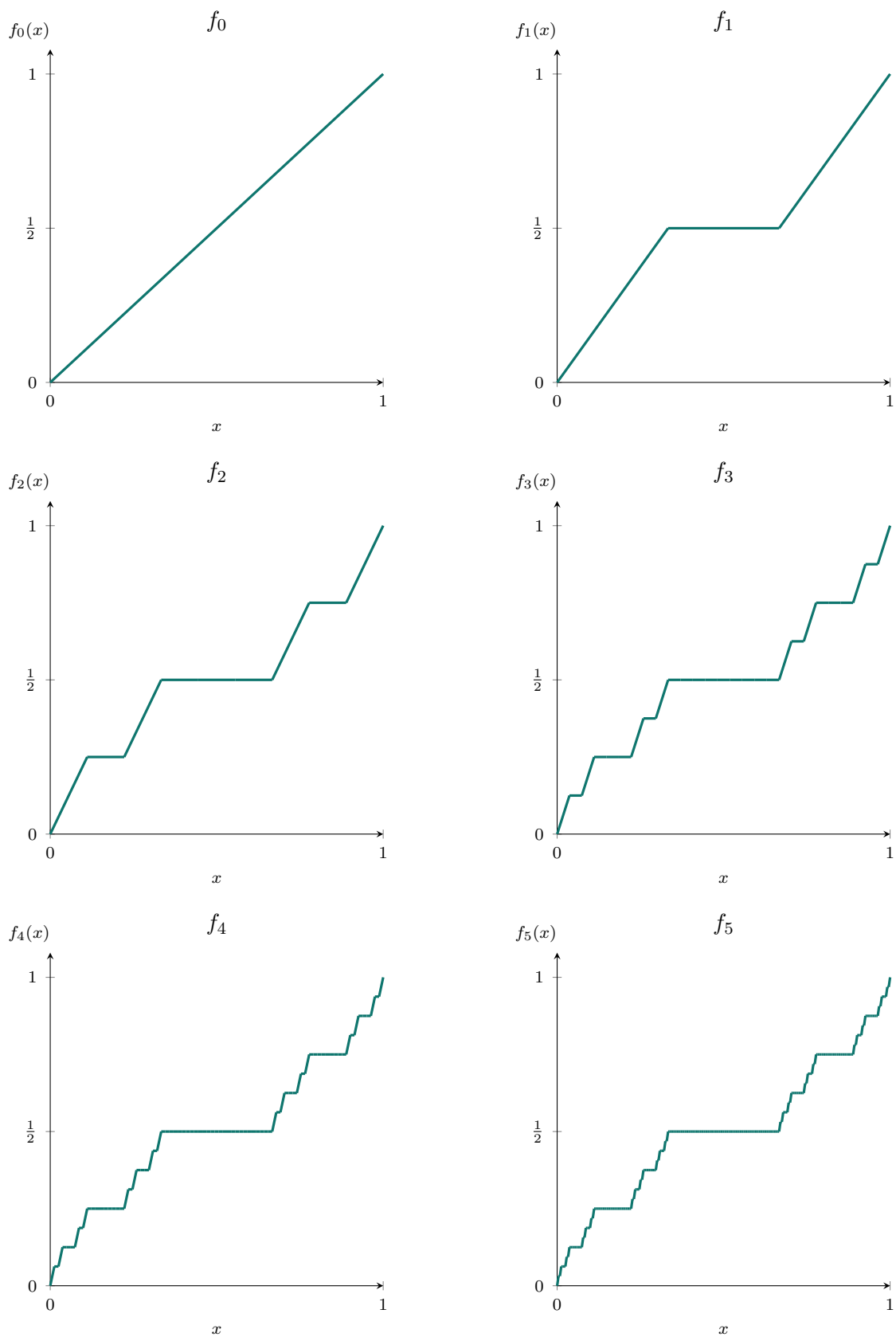
Figura 5: As primeiras seis aproximações da função de Cantor. O primeiro quadro corresponde a f_0 , e cada quadro seguinte é obtido do anterior pela regra descrita no texto; em cada etapa, o gráfico é achatado no terço médio de cada intervalo restante.
