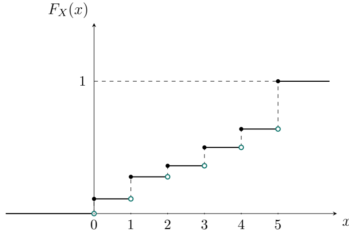
Figura 2: A função de distribuição de uma variável aleatória que assume valores no conjunto \{0, 1, 2, 3, 4, 5\} . O salto em x = 2 , por exemplo, é exatamente o valor de p_2 .
