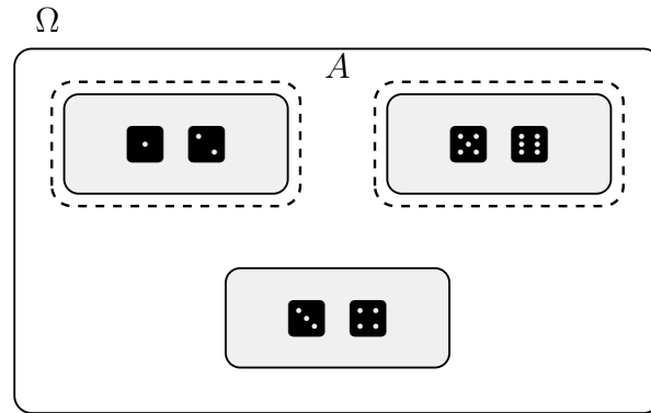
Figura 2: A \sigma -álgebra do Exemplo 5: os três blocos formam uma partição de \Omega , e cada evento é uma união de blocos. Em destaque, o evento A = \{\blacksquare, \blacksquare, \blacksquare, \blacksquare\} .
