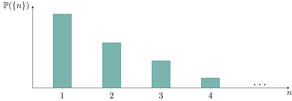
Figura 4: Diagrama ilustrando o valor da probabilidade de cada número natural segundo a função de probabilidade \mathbb{P}(\{n\}) = 6/\pi^2 n^2 definida pela função zeta do Exemplo 12 no caso s = 2 .
