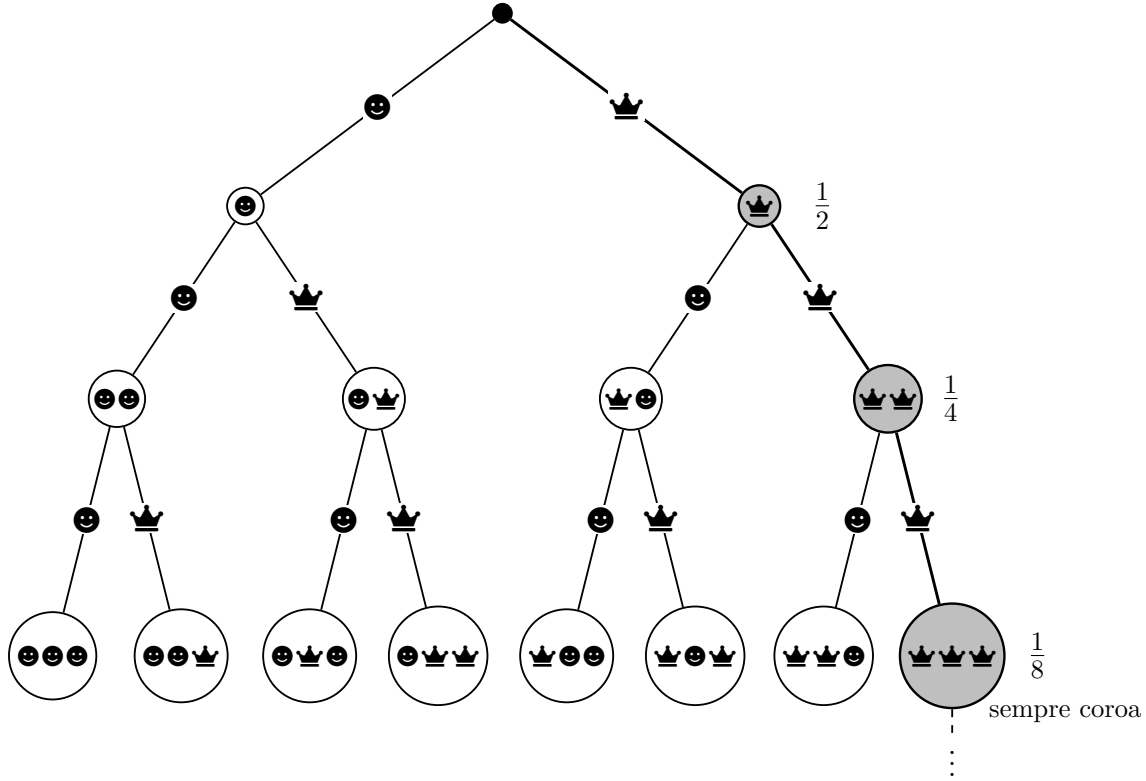
Figura 8: Os primeiros níveis da árvore de lançamentos do Exemplo 15 . O caminho destacado corresponde a nunca obter cara: a probabilidade de que os primeiros n lançamentos sejam todos coroa é 2^{-n} , que tende a 0 quando n \rightarrow \infty .
