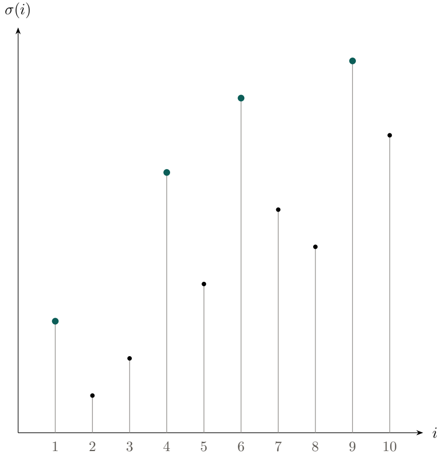
Figura 12: A permutação \sigma = (3, 1, 2, 7, 4, 9, 6, 5, 10, 8) vista como uma sequência de observações: os instantes 1, 4, 6 e 9, destacados, são recordes. Aqui R(\sigma) = 4 , um pouco acima do valor esperado H_{10} \approx 2,93 .
