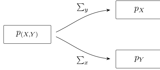
Figura 2: Obtenção das funções de probabilidade marginais a partir da função de probabilidade conjunta, somando sobre a coordenada complementar.
