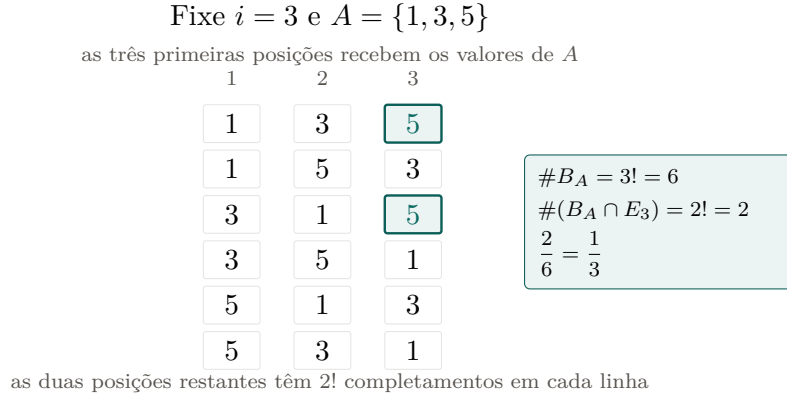
Figura 11: Dentro do bloco correspondente a A = \{1, 3, 5\} , há 3! ordens possíveis para as primeiras três posições. O recorde em i = 3 ocorre exatamente nas duas linhas em que o maior valor, 5, aparece na posição 3.
