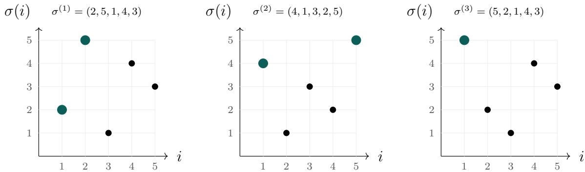
Figura 9: Três gráficos de funções discretas i \mapsto \sigma(i) para permutações de \{1, 2, 3, 4, 5\} . Cada linha e cada coluna contém exatamente um ponto. Os pontos em destaque são recordes; portanto, da esquerda para a direita, os números de recordes são 2, 2 e 1.
