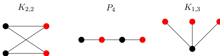
Figura 5: Três exemplos de grafos bipartidos.
